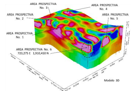
Método Magnetometría en 3D
