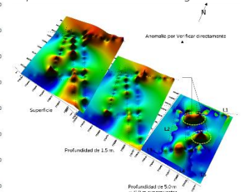
Cuerpo Mineralizados – Método Magnetometría
