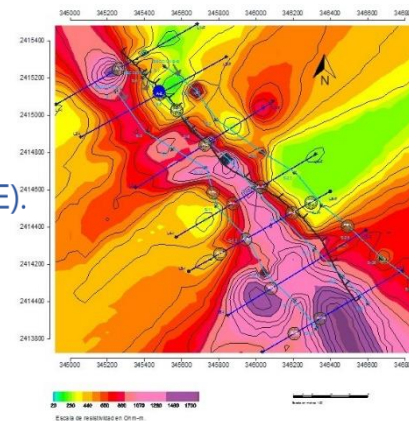
Método CSAMT
